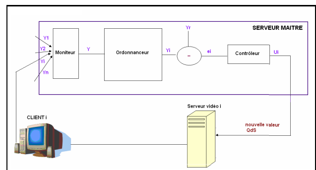
FIG. 2 – Architecture de contrôle par rétroaction de serveur maître.
