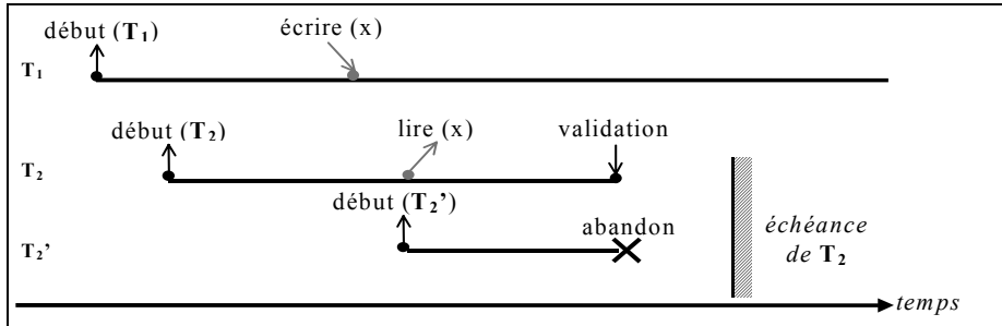
Figure 6. Ordonnement avec SCC-OB, en absence de conflit potentiel
