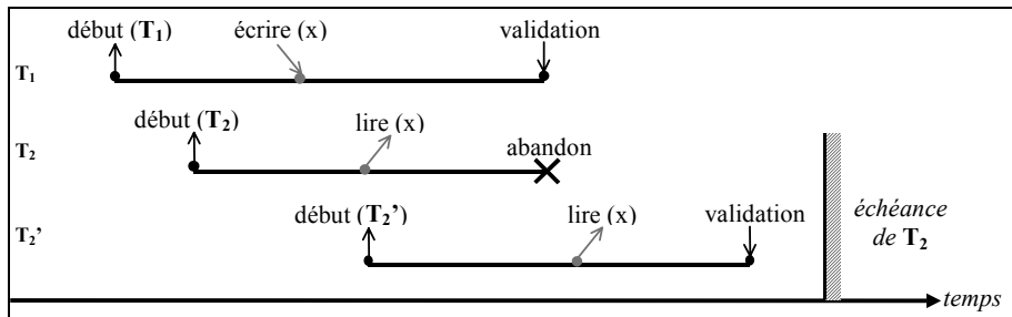
Figure 7. Ordonnement avec SCC-OB, en présence de conflit
