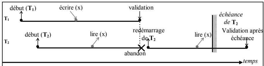
Figure 3. Ordonnement avec OCC-BC
